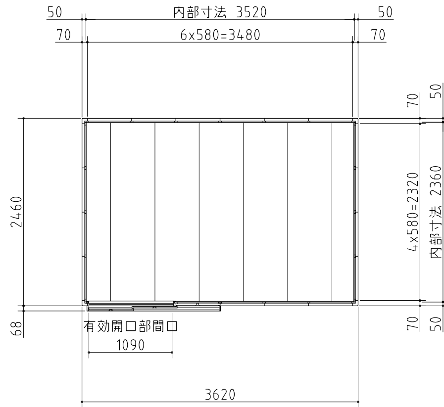
平面図
